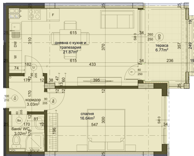
W-05 ВХОД "Б" АПАРТАМЕНТ 9 1:50
