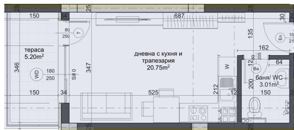
W-05 ВХОД "А" АПАРТАМЕНТ 15 1:50
